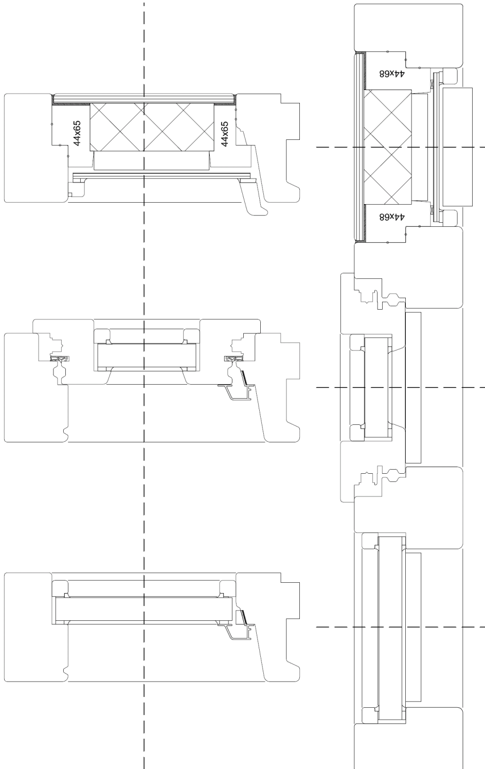
Bijlage 4 Variant voorzien van aluminium profiel op de onderdorpel
